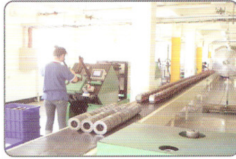
自動入線機 Stator coil & wedge inserter
